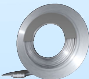
BALLIGE KAMMPROFILDICHTUNG MIT WEICH- STOFFAUFLAGE UND LOSEM ZENTRIERRING
