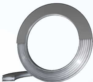
BALLIGE KAMMPROFILDICHTUNG FÜR FLANSCH MIT NUT UND FEDER
